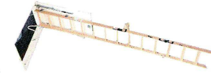
Scala retrattile modello 4 PEZZI LEGNO (h.280/300) senza corrimano Legno verniciata colore naturale
